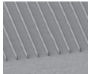
細小線寬/間距低至 15/15 \mu\text{m}
